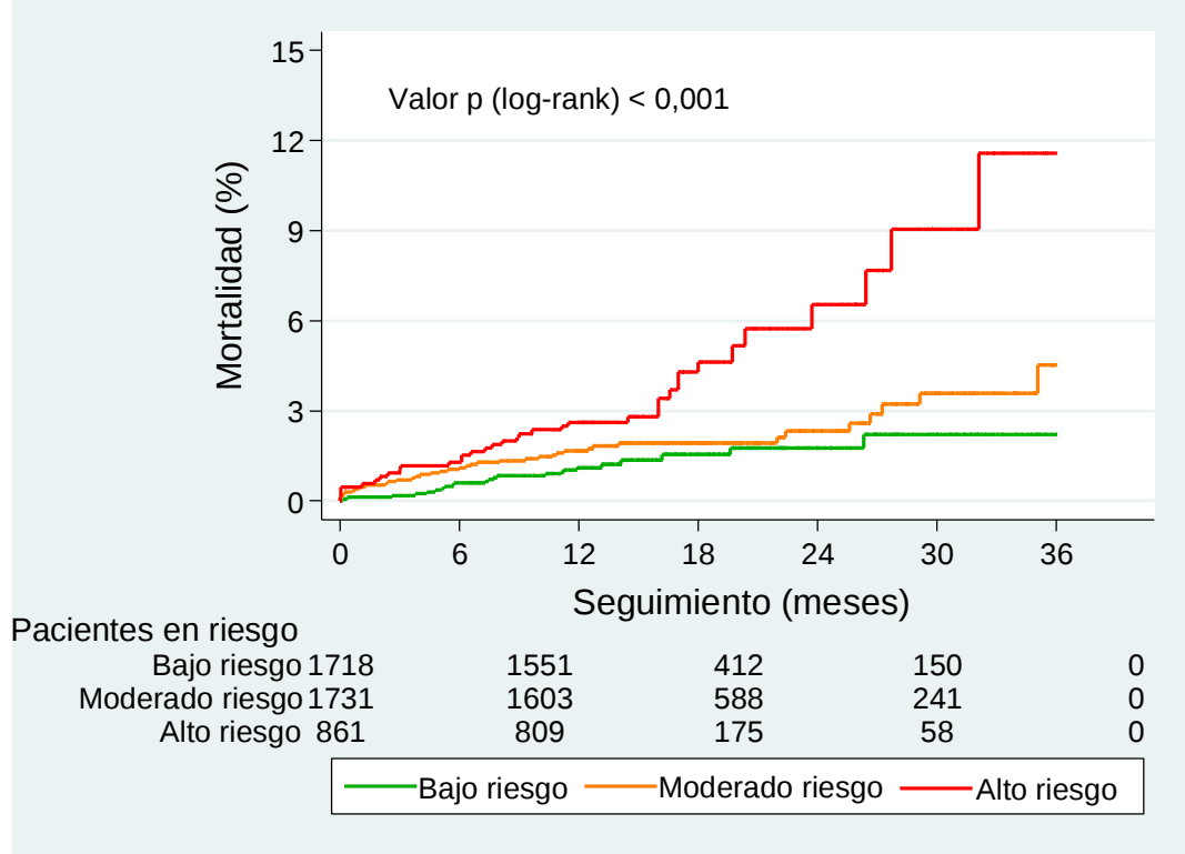
Figura 1 del material suplementario. Curvas de Kaplan-Meier de PARIS isquémico . Como variable continua, HR = 1,25 (IC95%, 1,08-1,45; p = 0,004); como variable categórica: moderado frente a bajo riesgo, HR = 1,46 (IC95%, 0,68-3,14; p = 0,329); alto frente a bajo riesgo, HR = 3,07 (IC95%, 1,76-5,35; p < 0,001). Estadístico C de Harrell de mortalidad, para PARIS isquémico . Como variable continua, C = 0,65 (IC95%, 0,61-0,69); como variable categórica, C = 0,63 (IC95%, 0,59-0,67). HR: hazard ratio ; IC95%: intervalo de confianza del 95%.
