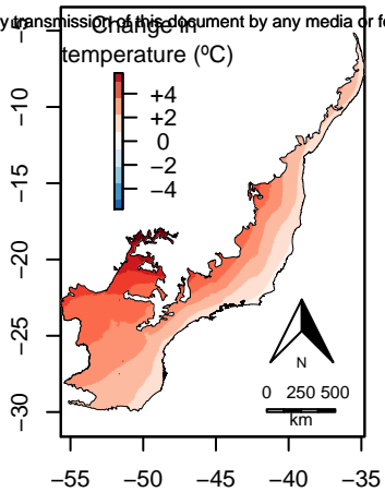
c) Temp. warmest quarter
